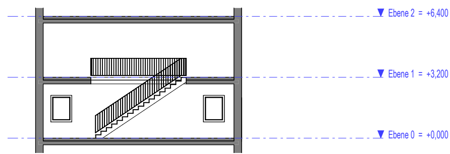
Schnitt A-A M 1:200
