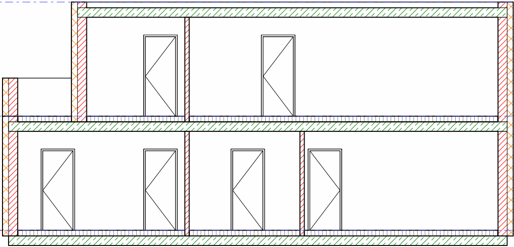
Schnitt s3 M 1:100
