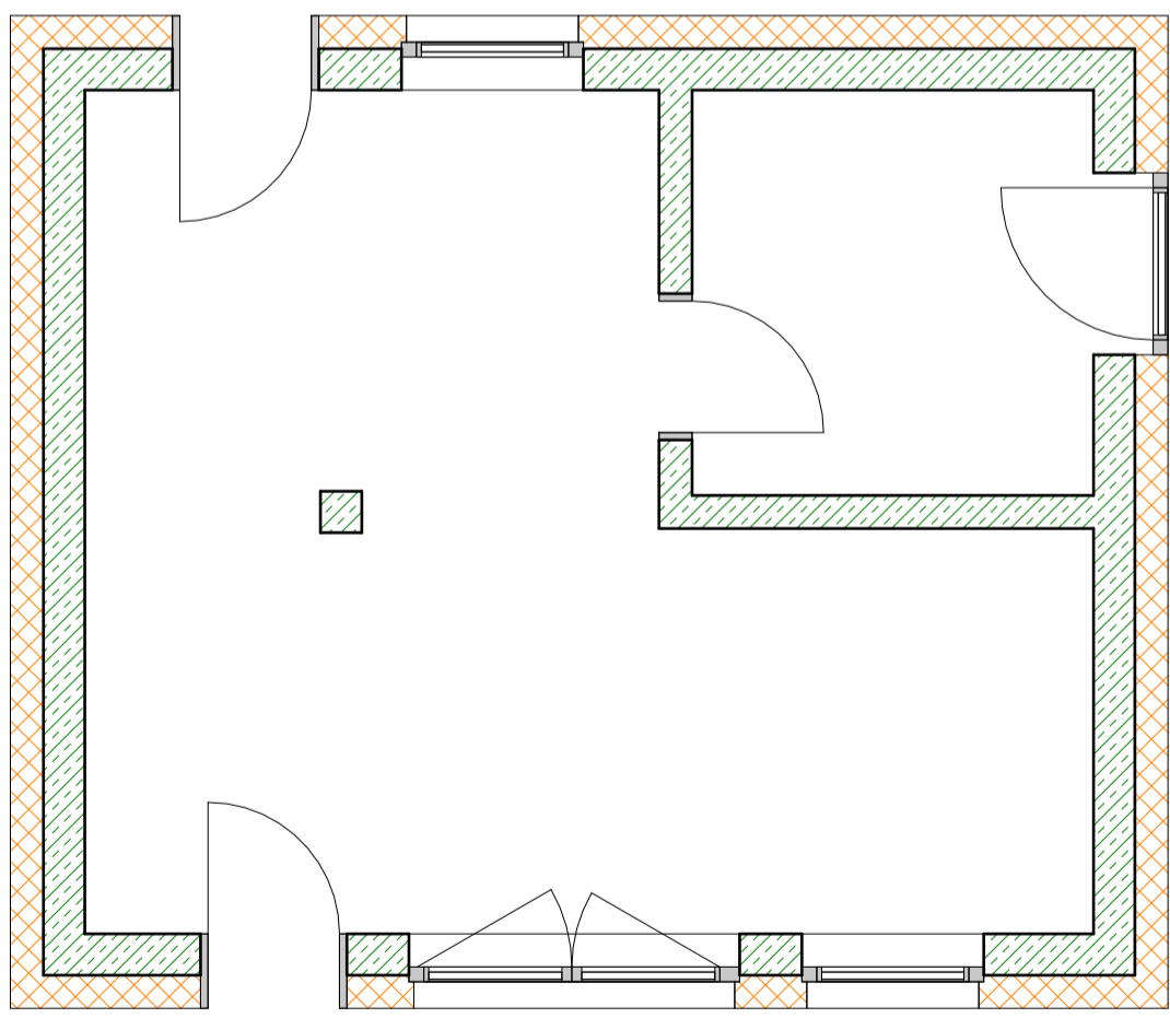
Grundriss; Detaillierungsgrad: mittel M 1 : 50
