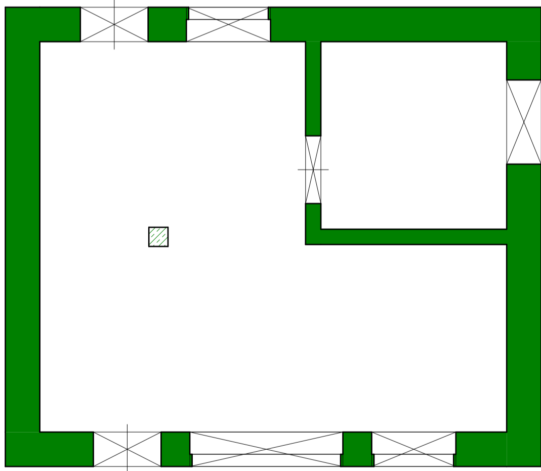
Grundriss; Detaillierungsgrad: grob M 1 : 50
