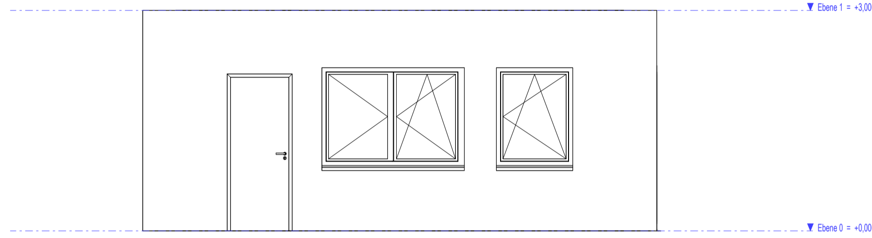
Süd Detaillierungsgrad fein R M 1 : 50
