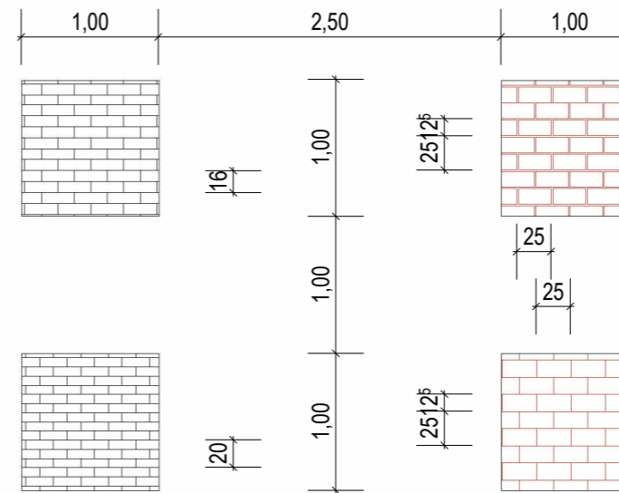
Darstellung Mauerwerk 0050 M 1 : 50
